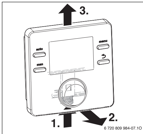
Мал. 8 Зняття пристрою
