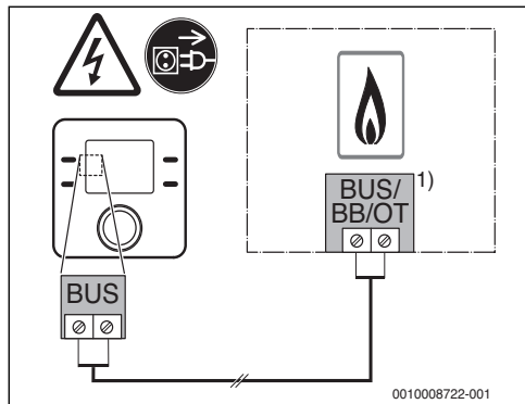
Мал. 6 Підключення пристрою керування до теплогенератора
